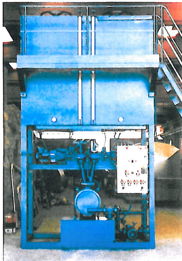
fig 3 IMPIANTI PER LA PRODUZIONE DI EMULSIONI BITUMINOSE.
